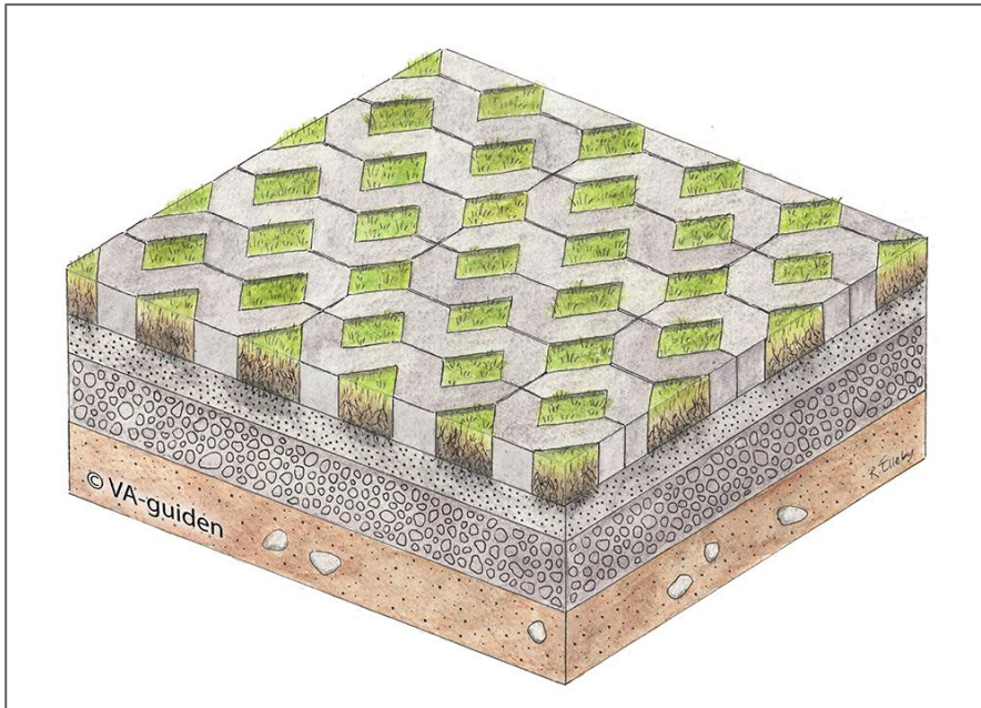
Figur 18. Illustrationskiss som visar uppbyggnaden av permeabel beläggning. Skiss: VA-guiden, 2024
